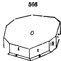
Binnenthal.
